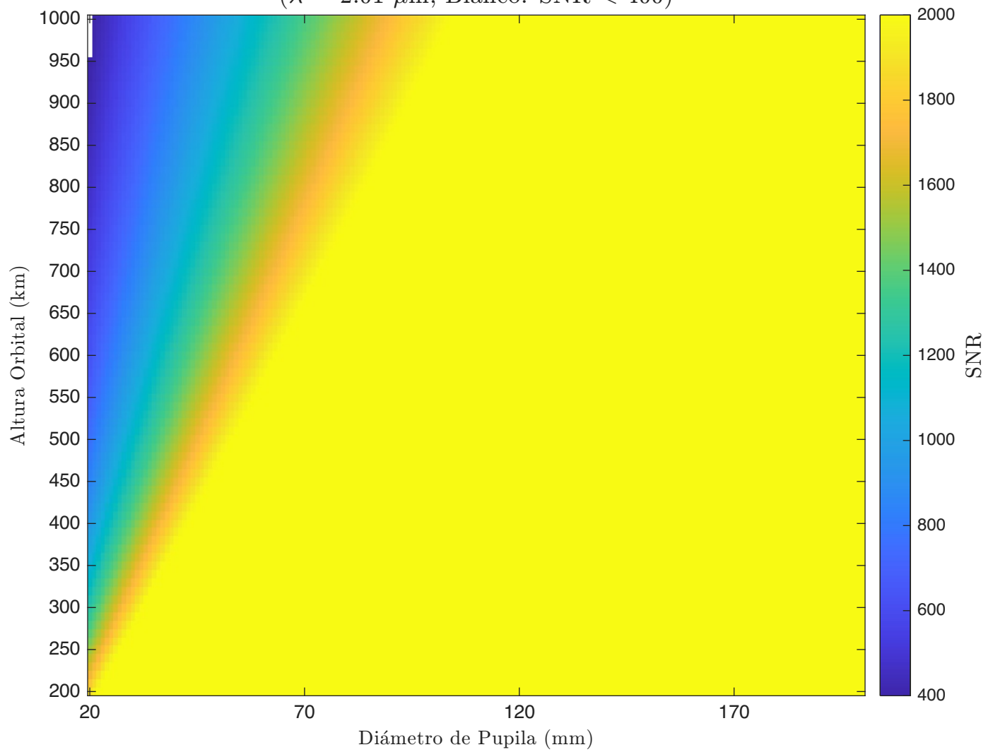
SNR - Korsch - Detector 2 ( \lambda = 2.01 \mu\text{m} , Blanco: SNR < 400)
